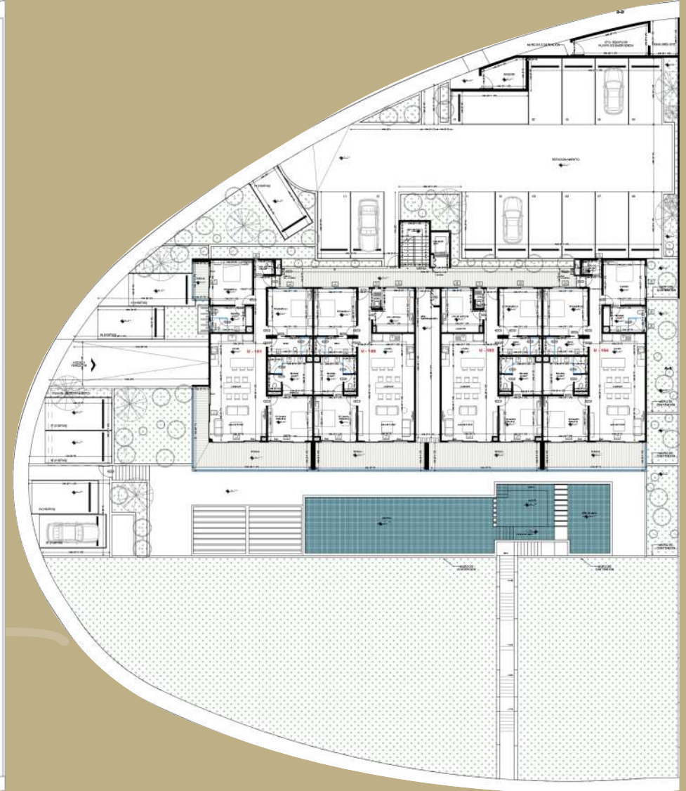
Architectural plant 1st level Planta arquitectónica 1er nivel
