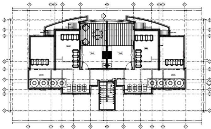
PLANTA ARQUITECTÓNICA N-A 179.828 m²
